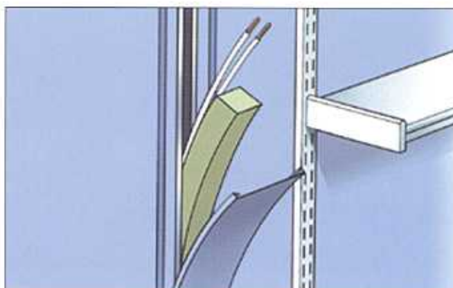
Elledningarna är infällda i väggfogarna. Vägghkonstruktion: Brännlackerad stålplåt på ömse sidor om gipsförstyvning och obrännbar isolering.
